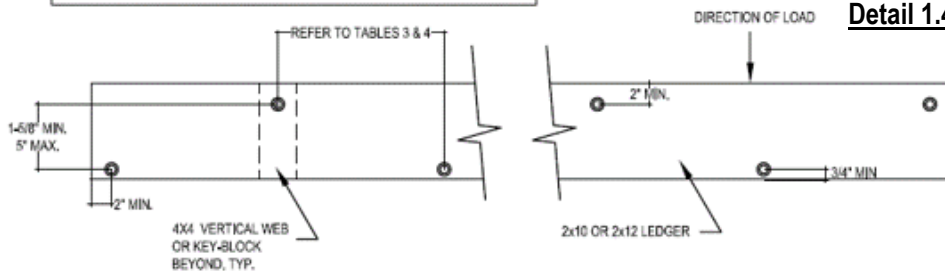
Detail 1.4
